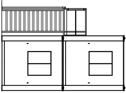
RIGHT ELEVATION
